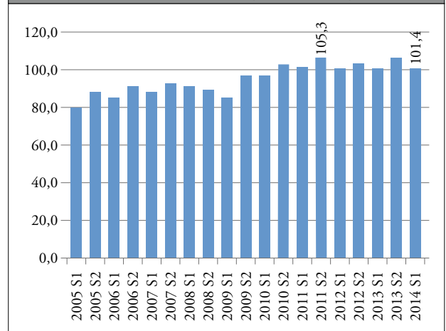
Grafik 1: Türkiye Çalışılan Saat Başına Üretim Endeksi (2010=100)
