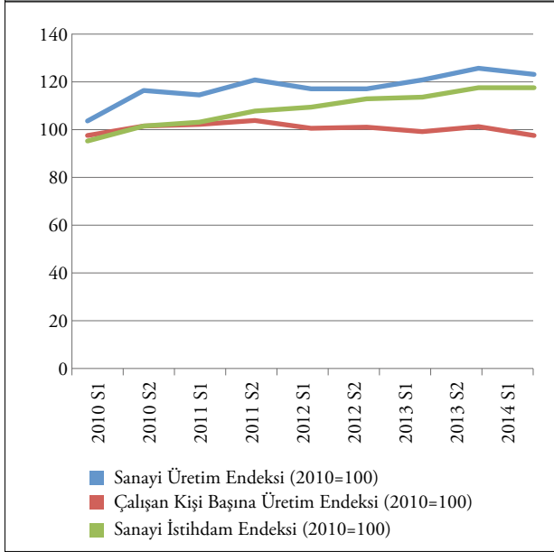
Grafik 2: Türkiye 2010-2014 Sanayi Üretimi, İstihdam ve Verimlilik
